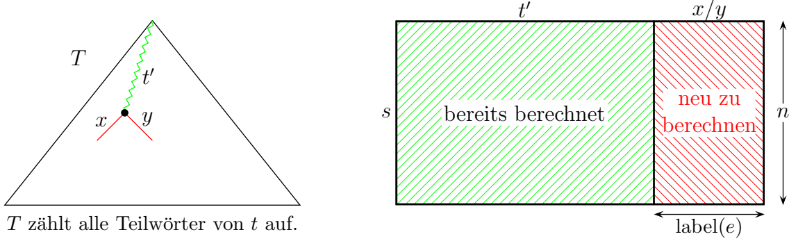
Abbildung 4.41: Skizze: Hybrides Verfahren für One-Against-All
