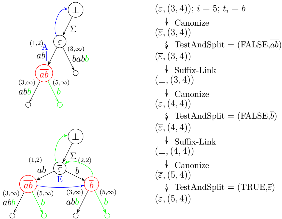
Abbildung 3.25: Beispiel: Ukkonens Algorithmus: \hat{T}^5
