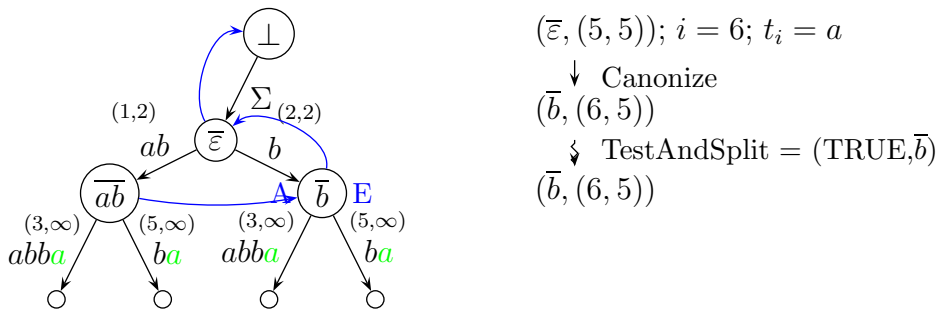
Abbildung 3.26: Beispiel: Ukkonens Algorithmus: \hat{T}^6
