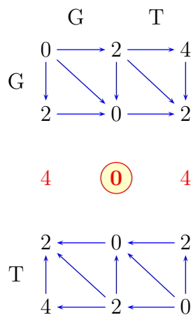
Abbildung 4.23: Beispiel: Zweiter rekursiver Aufruf im Hirschberg-Algorithmus
