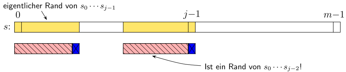
Abbildung 2.7: Skizze: Das um ein Zeichen kürzere Präfix des eigentlichen Randes von s_0 \dots s_{j-1} ist ein Rand von s_0 \dots s_{j-2}
