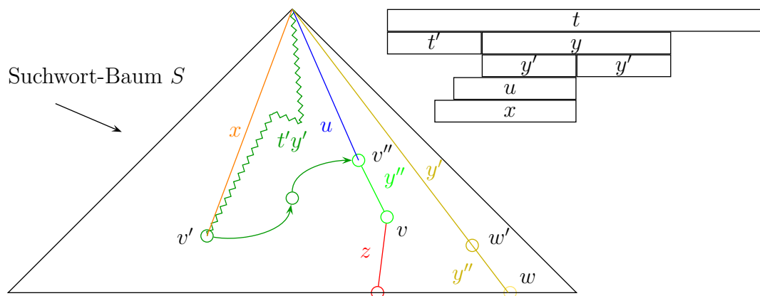
Abbildung 2.19: Skizze: Im Suchwort-Baum wird Treffer von y gemeldet
