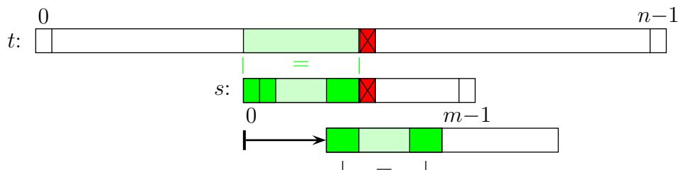
Abbildung 2.4: Skizze: Eine Idee für größere Shifts
