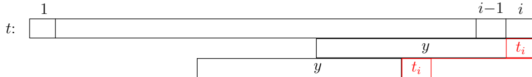
Abbildung 3.13: Skizze: Vom Endknoten von T^{i-1} zum aktiven Knoten von T^i
