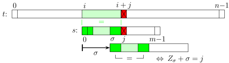
Abbildung 2.46: Skizze: Shift bei KMP
