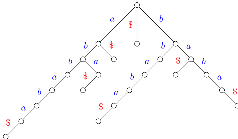
Abbildung 3.2: Beispiel: t = abbaba\$
