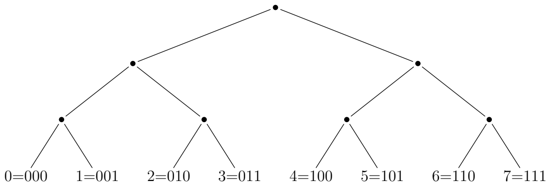
Abbildung 6.22: Skizze: Nummerierung der Blattsequenzen
