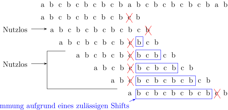
Abbildung 2.21: Beispiel: Suchen mit der zweiten naiven Methode
