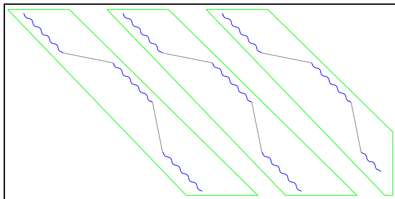
Abbildung 6.27: Skizze: Optimale Alignments um die Pfade aus Diagonal Runs
