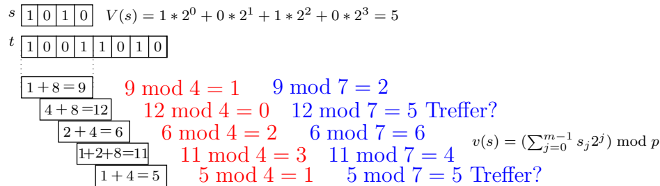
Abbildung 2.48: Beispiel: Numerische Suche von 1010 in 10011010 modulo 7
