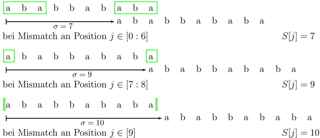
Abbildung 2.28: Beispiel: s = ababbababa (Teil 2: \sigma > j )
