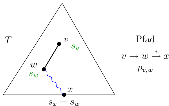
Abbildung 6.15: Skizze: Kante (v, w) definiert mithilfe von T einen Pfad p_{v,w} in T
