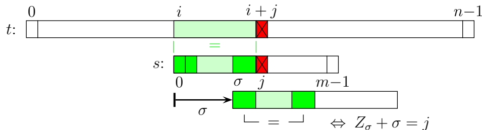
Abbildung 2.42: Skizze: Shift bei KMP
