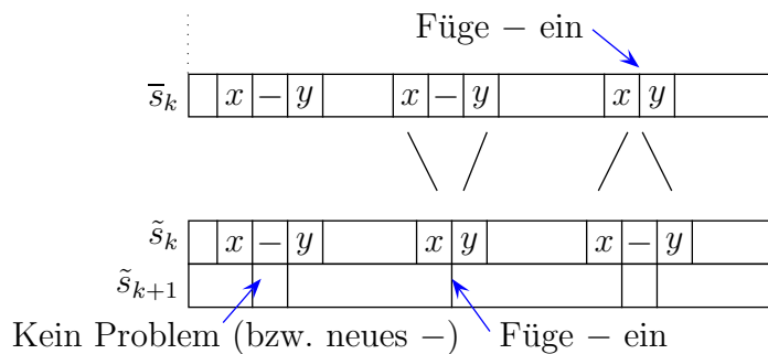
Abbildung 6.11: Skizze: Erweiterung des mehrfachen Sequenzen-Alignments
