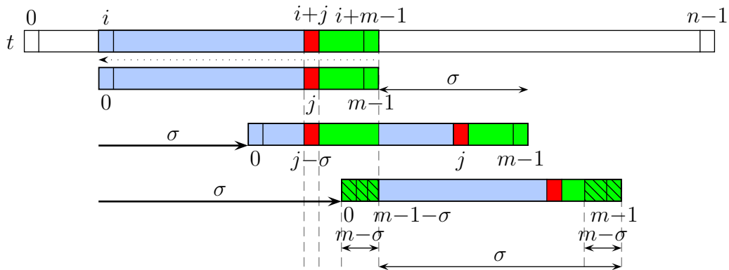
Abbildung 2.22: Skizze: Zulässige Shifts bei Boyer-Moore (Strong-Good-Suffix-Rule)
