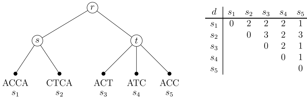
Abbildung 6.19: Beispiel: Dynamische Programmierung für geliftetes PMSA
