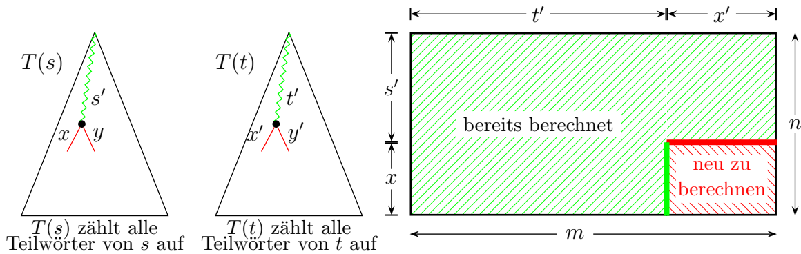
Abbildung 4.42: Skizze: Hybrides Verfahren für All-Against-All
