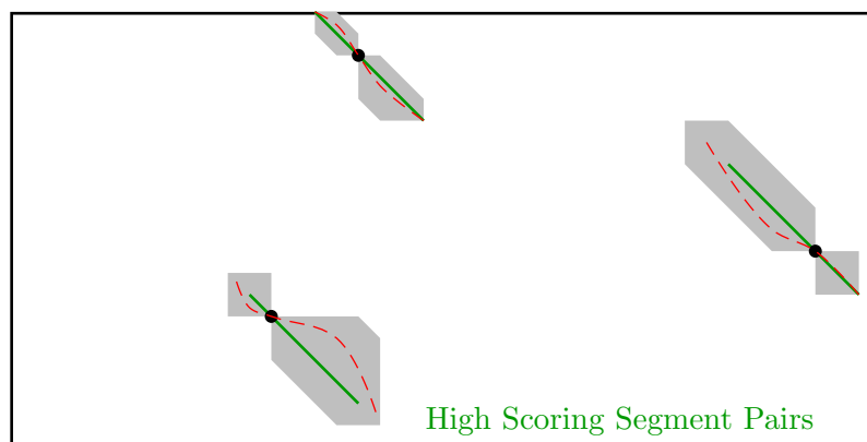
Abbildung 6.31: Skizze: Erweiterung der High Scoring Segment Pairs
