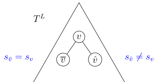
Abbildung 6.21: Skizze: Bild zur Notation der gelifteten Kindsequenzen
