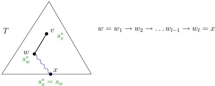
Abbildung 6.16: Skizze: Pfad p_{v,w} im optimalen Baum (T, \varphi^*)
