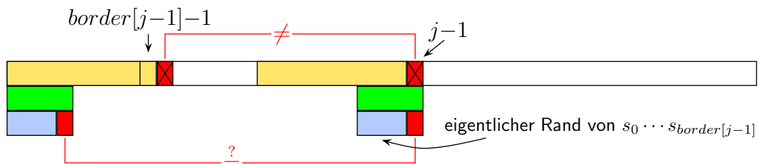
Abbildung 2.8: Skizze: Berechnung von border[j] durch Verlängerung eines Randes
