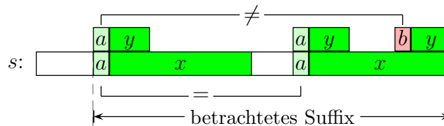
Abbildung 2.26: Skizze: Nichtbeachtung der Verlängerung kürzerer Ränder eines Suffixes
