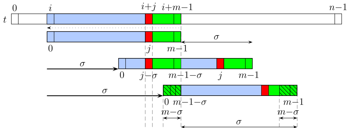
Abbildung 2.44: Skizze: Zulässige Shifts bei Boyer-Moore (Strong-Good-Suffix-Rule)
