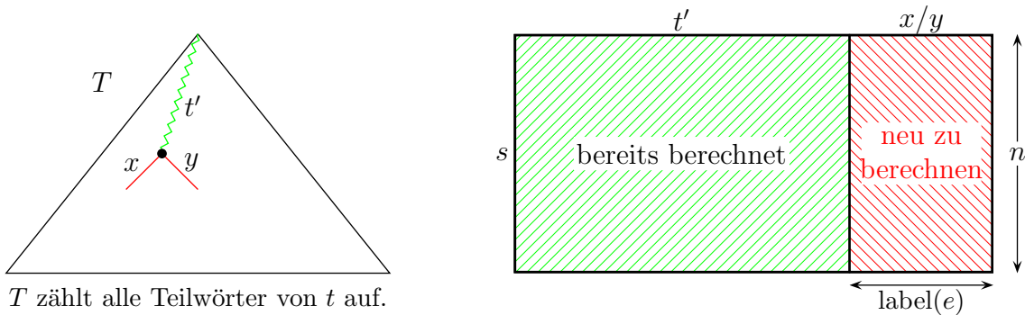
Abbildung 4.40: Skizze: Hybrides Verfahren für One-Against-All
