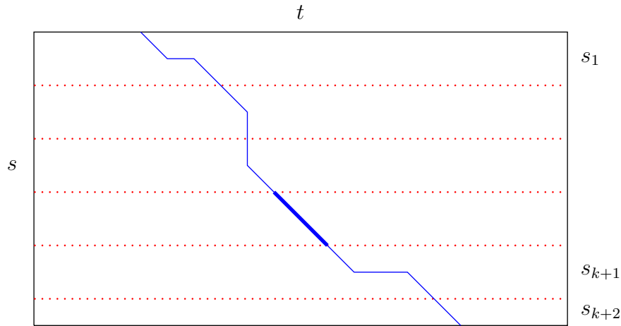
Abbildung 6.32: Skizze: Alignment mit Editdistanz k = 4
