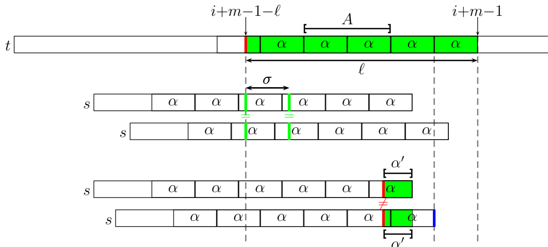
Abbildung 2.32: Skizze: Mögliche frühere initiale Vergleich im Bereich A
