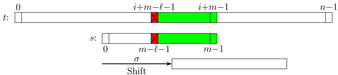
Abbildung 2.30: Skizze: Shift nach \ell erfolgreichen Vergleichen
