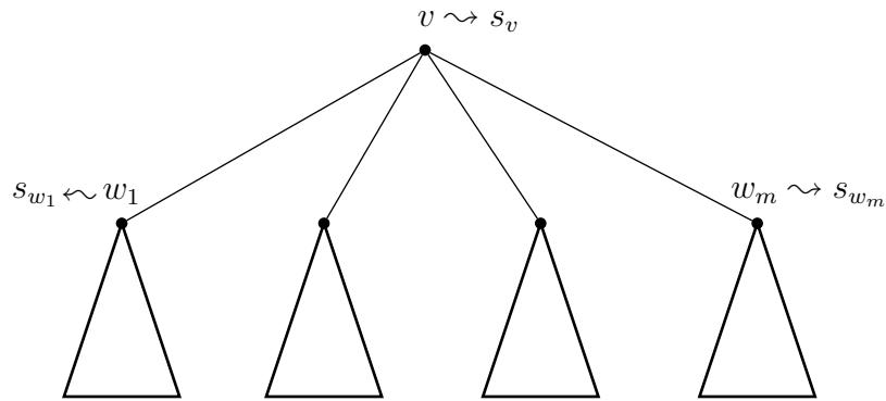
Abbildung 6.18: Skizze: Berechnung von D(v, s)
