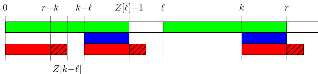
Abbildung 2.39: Skizze: Fall 2b
