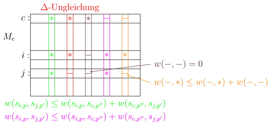
Abbildung 6.12: Skizze: Beweis der Dreiecksungleichung
