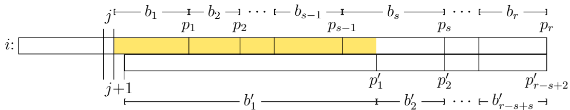
Abbildung 4.39: Skizze: Veränderung der Blockstruktur
