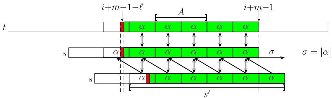
Abbildung 2.31: Skizze: Periodisches Ende von s bei kurzen Shifts
