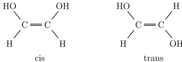
Abbildung 10: Skizze: Cis-Trans-Isomerie bei Äthendiol
