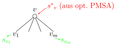
Abbildung 6.14: Skizze: Liften eines Knotens
