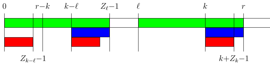
Abbildung 2.38: Skizze: Fall 2a
