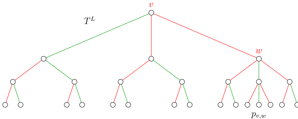
Abbildung 6.17: Skizze: Beziehung Kantengewichte in T^L zu T^*
