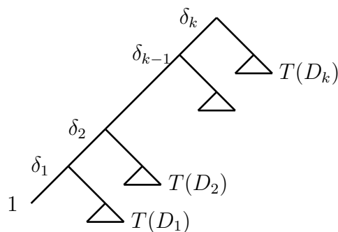
Abbildung 2.23: Skizze: Rekursive Konstruktion ultrametrischer Bäume
