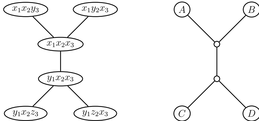
Abbildung 2.19: Beispiel: Baumzerlegung in Cliques und zugehöriger phylogenetischer Baum
