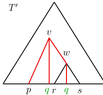
Abbildung 2.40: Skizze: Kante (v, w) in T'
