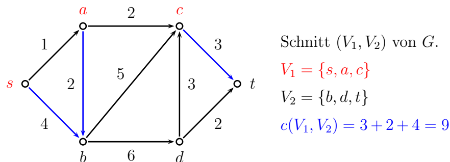
Abbildung 3.2: Beispiel: Schnitt eines Graphen
