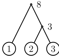
Abbildung 2.38: Gegenbeispiel: D nicht additiv, aber D' ultrametrisch
