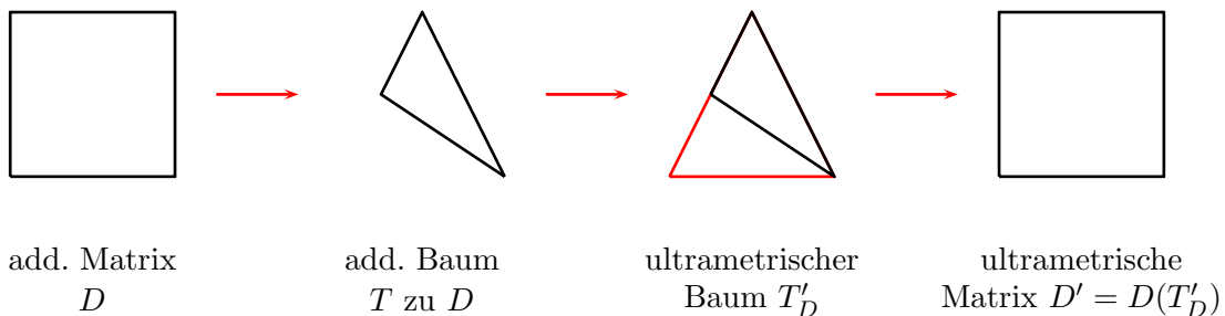
Abbildung 2.33: Skizze: Schema der Transformation einer additiven Matrix in eine ultrametrische Matrix
