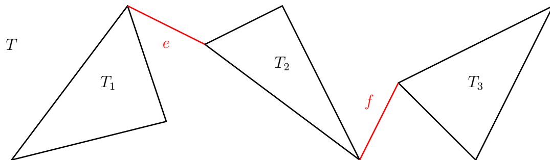
Abbildung 2.82: Skizze: Splits in T
